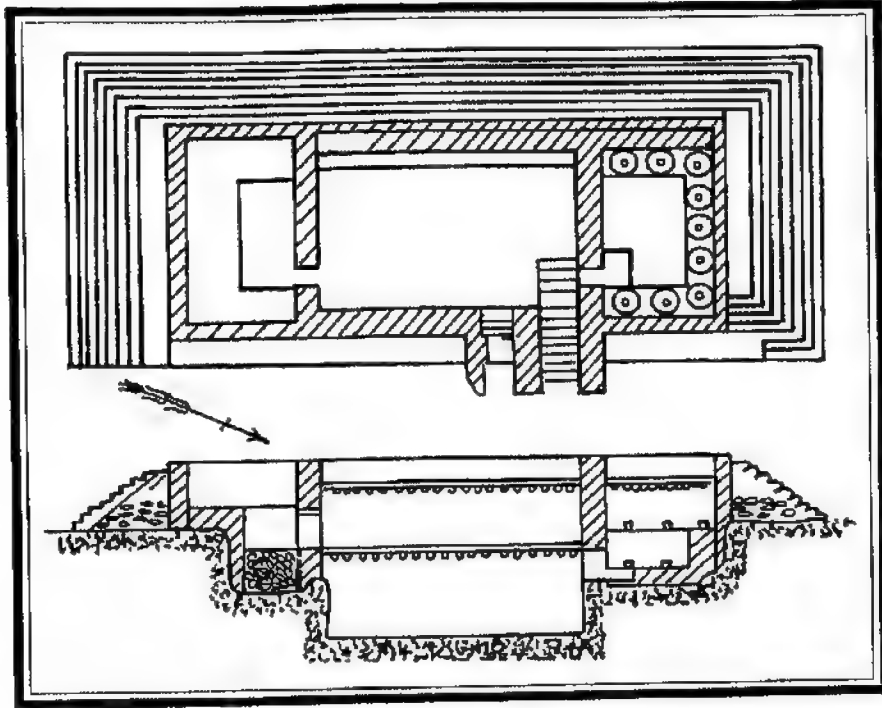
(شكل ٤٢) مسقطان أفقى ورأسى للمقبرة ٣٠٣٨ فى سقارة.
